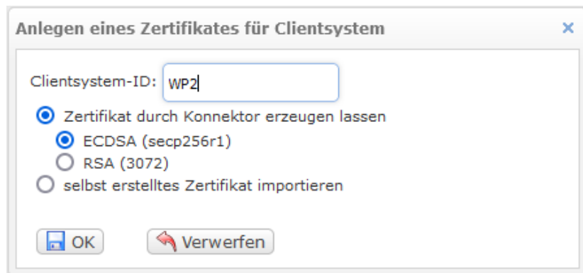
Abbildung 73: Konfiguration zum Anlegen eines Clientsystem-Zertifikats mit ECC
