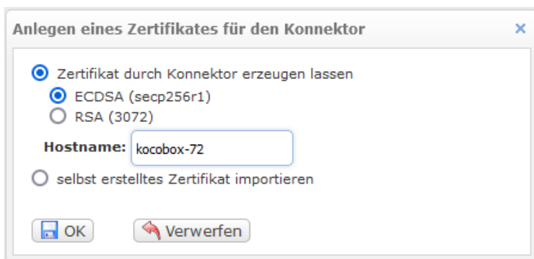
Abbildung 74: Anlegen eines Konnektor-Authentisierungszertifikats
