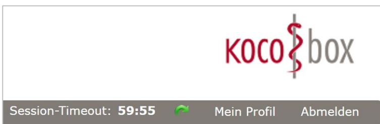
Abbildung 41: Session-Timeout zurücksetzen
