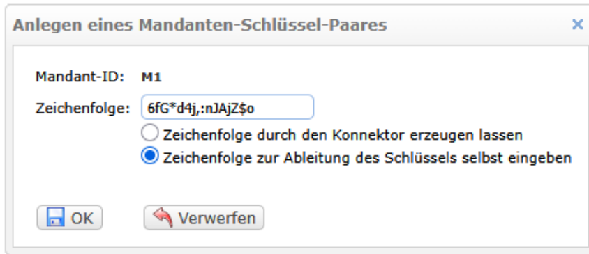
Abbildung 130: Konfigurationsfenster für das Anlegen eines Mandanten-Schlüssel-Paares
