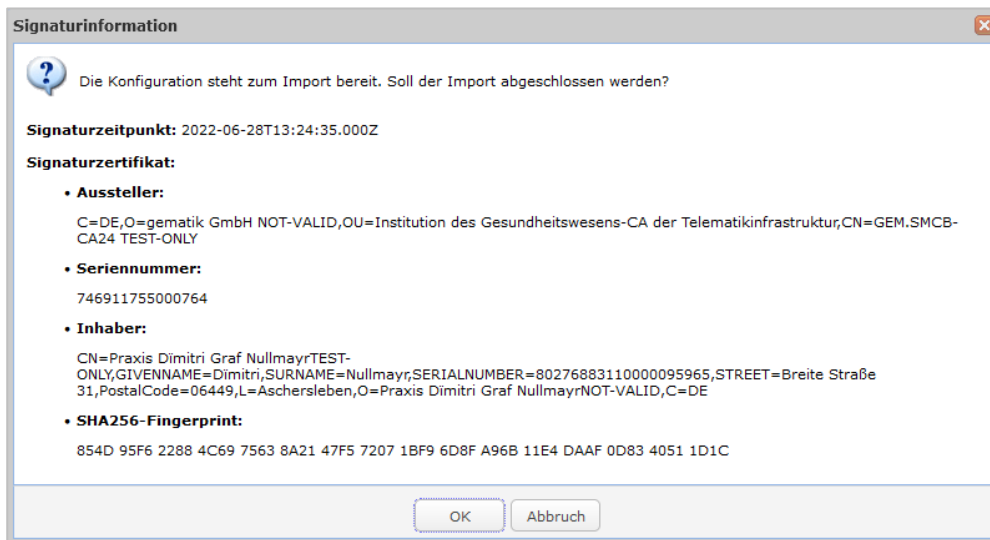
Abbildung 82: Anzeigefenster zur Kontrolle der Signaturinformationen
