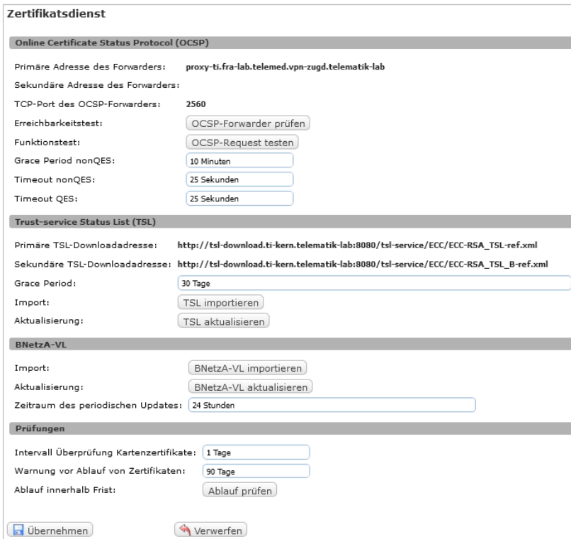
Abbildung 37: Konfigurationsbereich für den Zertifikatsdienst
