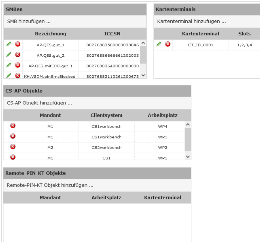
Abbildung 54: Infomodell-Konfigurationsbereiche für SMBen, Kartenterminals und CS-AP Objekte
