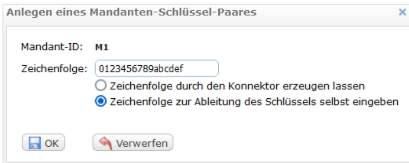
Abbildung 65: Konfigurationsfenster für das Anlegen eines Mandaten-Schlüssel-Paares
