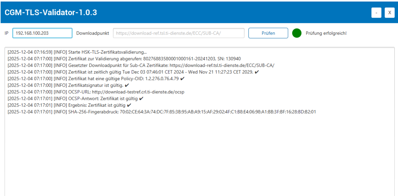
Abbildung 1: Beispiel für eine erfolgreiche Zertifikatsprüfung mittels TLS-Validator
