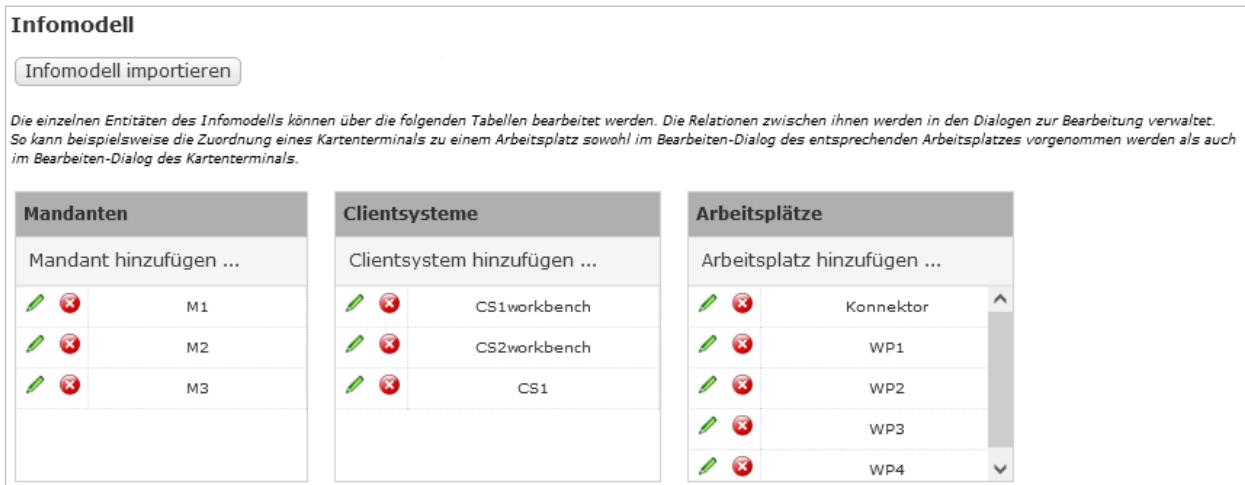
Abbildung 53: Infomodell-Konfigurationsbereiche für Mandanten, Clientsysteme und Arbeitsplätze
